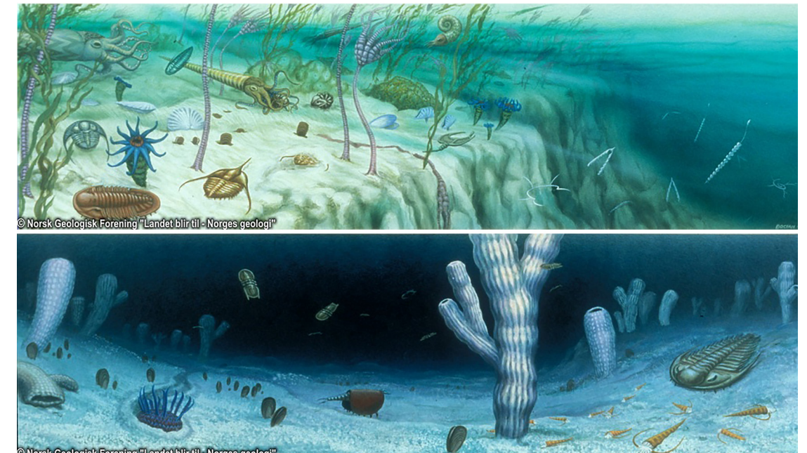
Figur 3: Slik kan havbunnen ha sett ut i jordas tidlige Oldtid. Skissen er fra boken «Landet blir til» utgitt av Norsk Geologisk Forening
