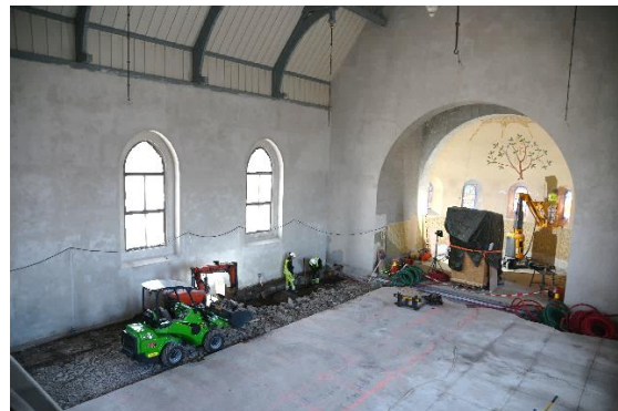
April 2020: Grøfter til energibrønner og varmeanlegg er lagt ned til uthuset, som skal bygges om til teknisk rom og lager.
