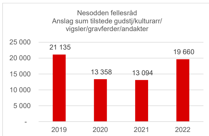
Figur 1: Beregnede gjennomsnittstall utarbeidet av Borg bispedømme, basert på SSB-tall
