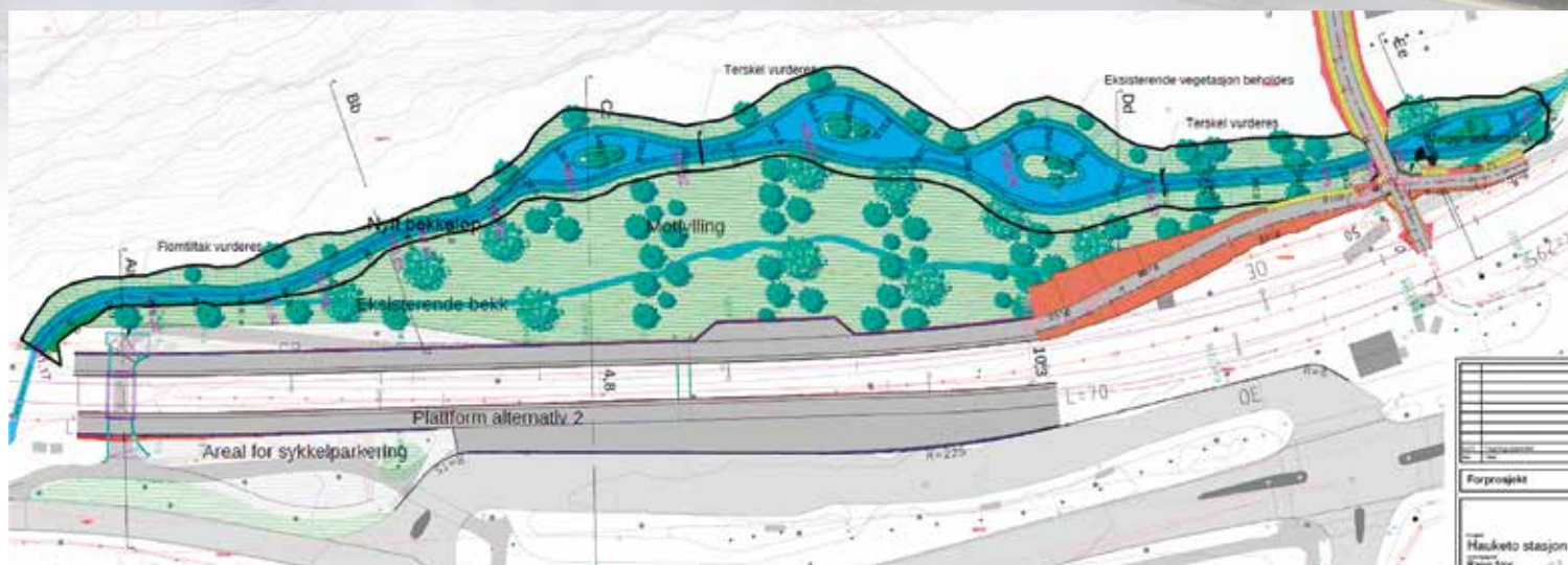
Kilde: Omlegging av bekkeløp, plan- og lengdeprofil, Bane NOR og Asplan Viak
