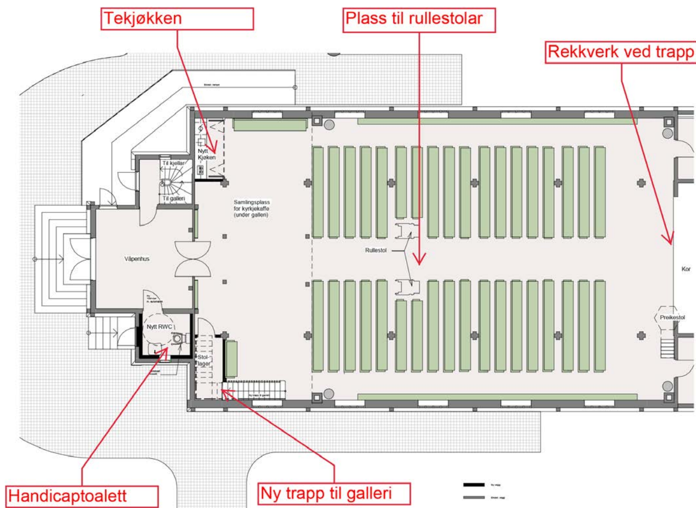
Teikninga viser handicaptaolett som kjem der trapp til galleriet er no, ny trapp, plassering av tekjøkken og utviding av midtgangen. Teikning: Arki arkitektar AS.
